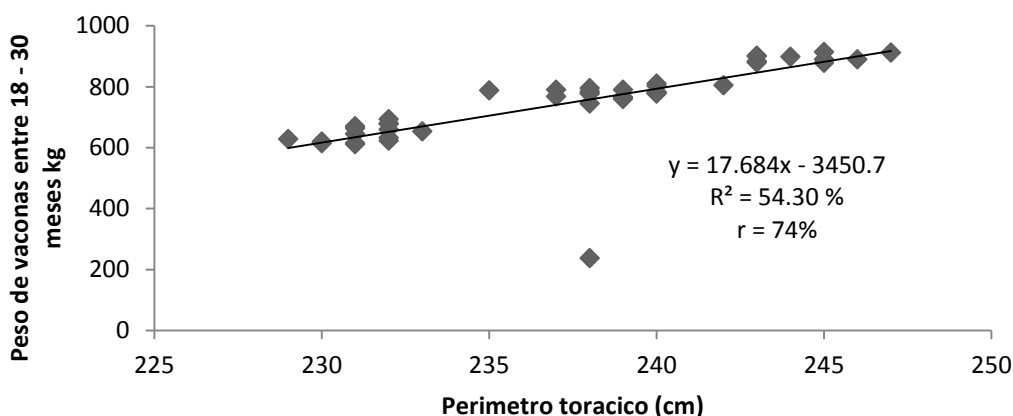
Grafico 62. Línea de tendencia entre el peso y el perímetro torácico de las hembras charoláis
