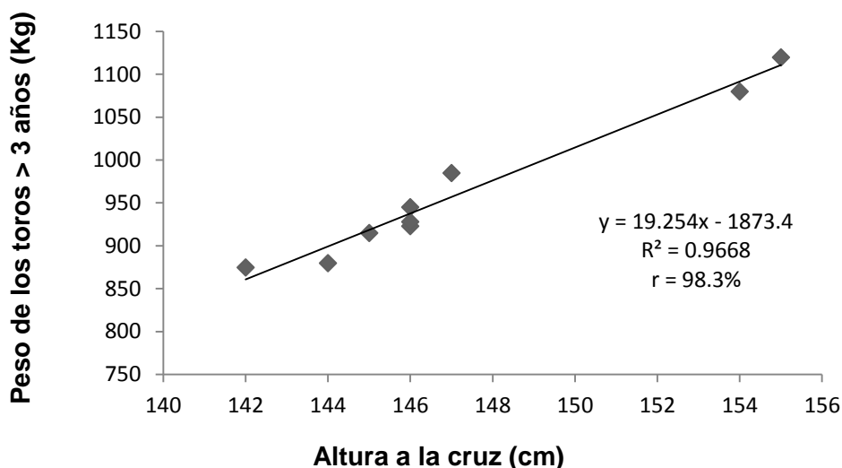
Grafico 5. Línea de tendencia entre el peso y la altura a la cruz de los toros charoláis mayores a 3 años
