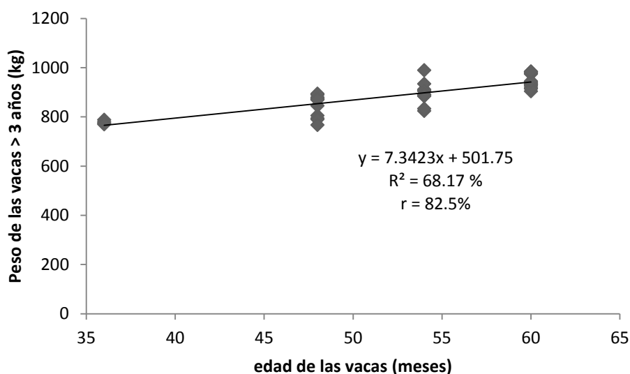
Gráfico 41. Línea de tendencia entre el peso y la edad de las hembras charoláis mayores a 30 meses de edad
