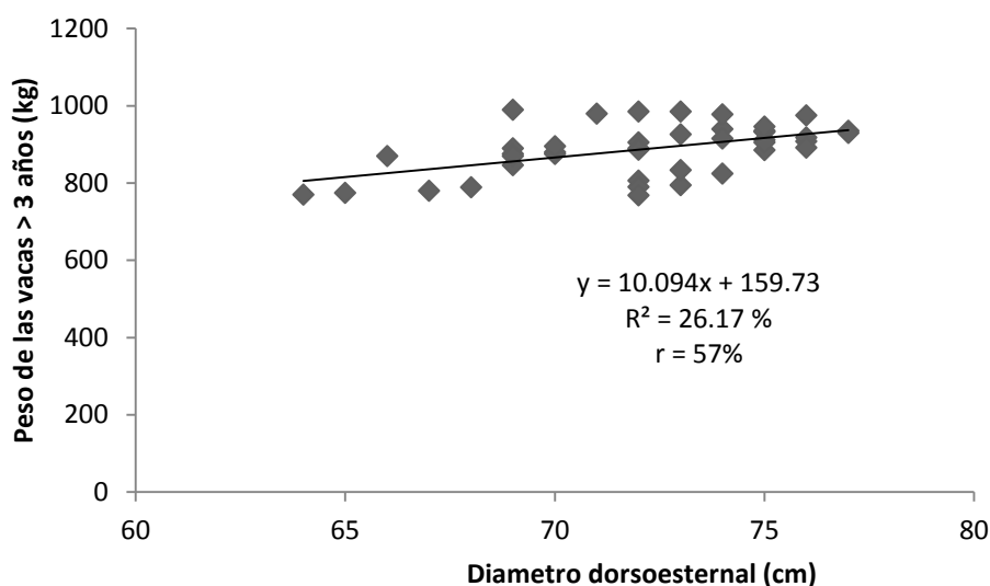
Grafico 47. Línea de tendencia entre el peso y el diámetro dorso esternal en hembras charoláis mayores a 30 meses de edad
