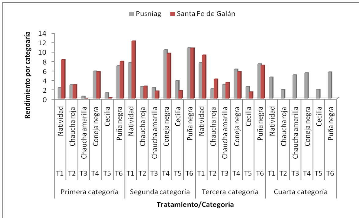
GRÁFICO 6. RENDIMIENTO POR CATEGORÍAS DE SEIS CULTIVARES DE PAPA EN PUSNIAG Y SANTA FE DE GALÁN.
