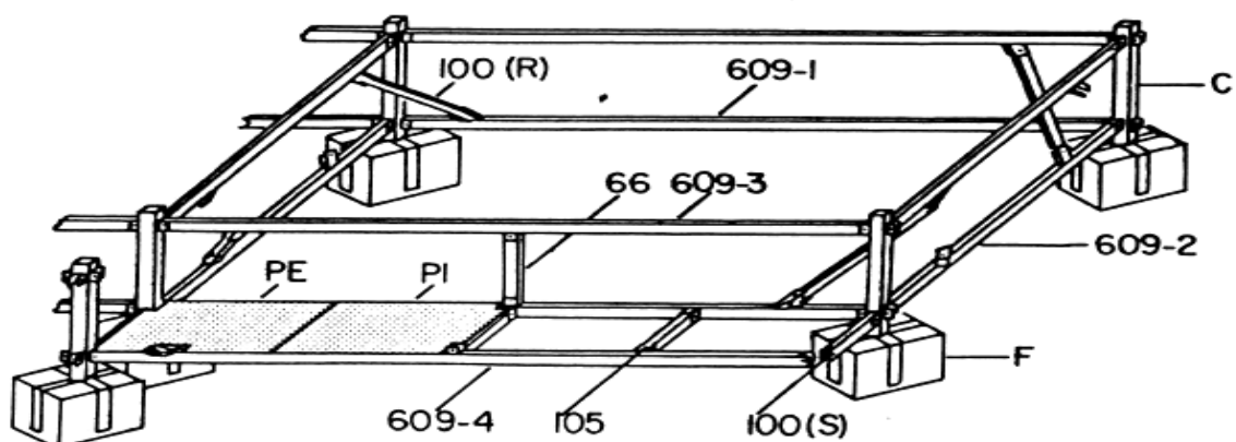
Gráfico 2. Diagrama de una jaula para siembra de alevines
