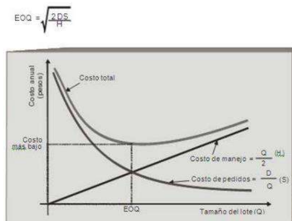
Figura 1-1: El modelo clásico EOQ
